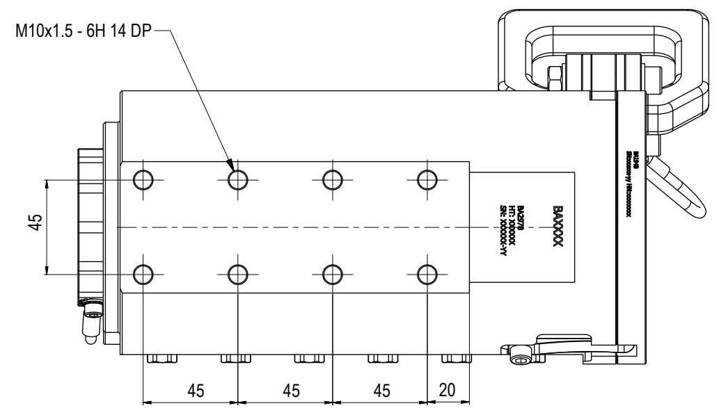
VIEW A-A
